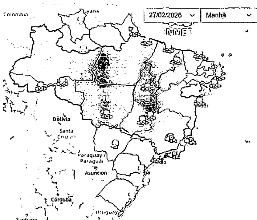
Figura 3: Previsão do Tempo: Fonte https://portal.inmet.gov.br/
